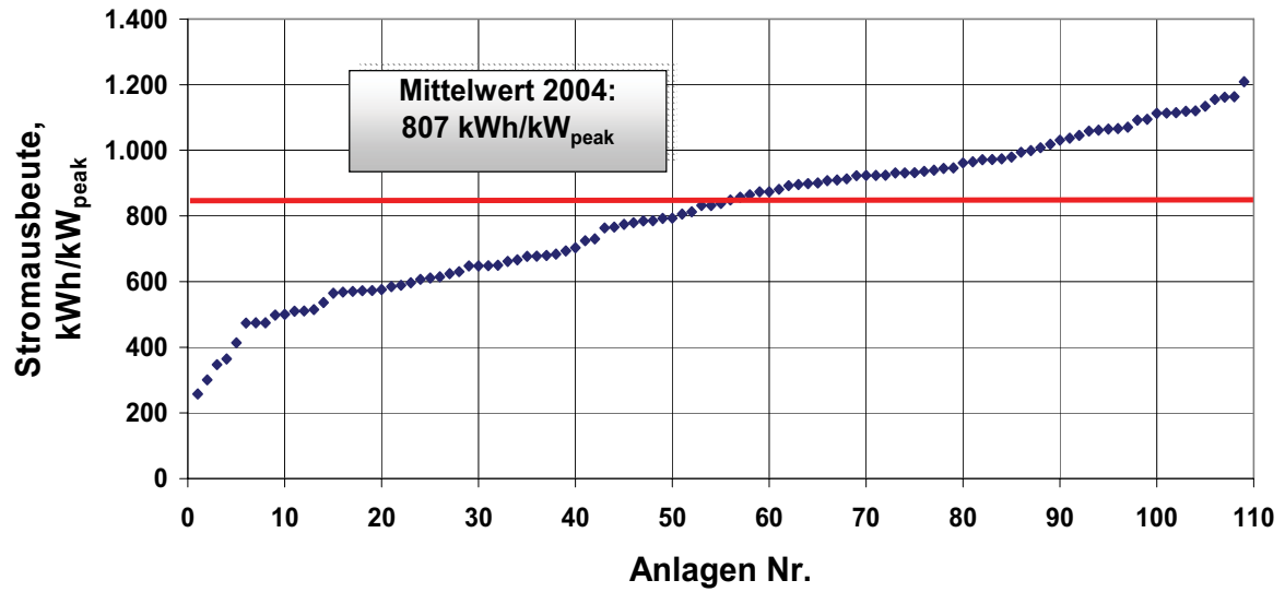
Abb. 19: Spezifischer Stromertrag von Netzgekoppelten PV-Anlagen in Österreich (Quelle: oekostrom AG und arsenal research)
