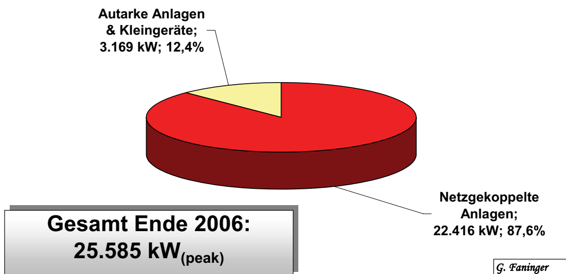
Abb. 9: Ende 2006 in Österreich installierte Photovoltaik-Anlagen Netzgekoppelte und autarke PV-Anlagen (Nach Firmenmeldungen)
