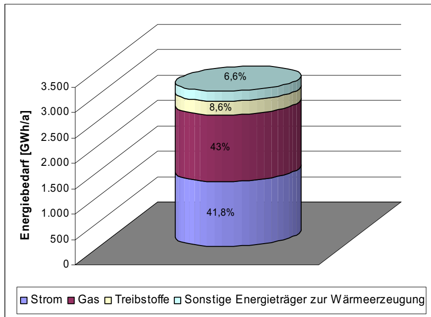
Abbildung 18: Anteil der betrachteten Energieträger am energetischen Endverbrauch in der Industrieregion im Jahr 2005 [Beteiligte Firmen]
