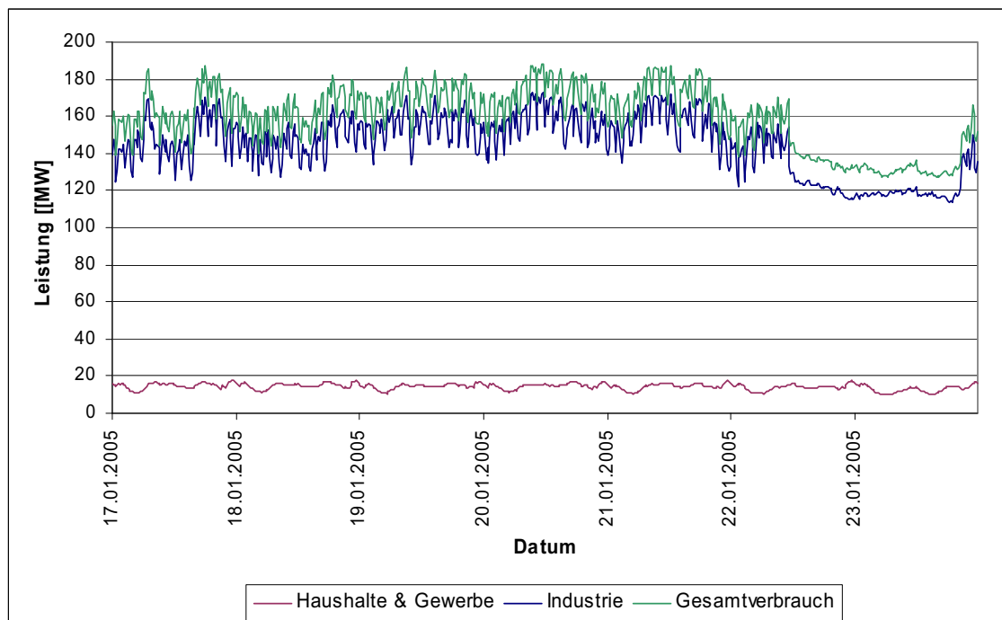
Abbildung 7: Leistungswerte des Stromverbrauches der 3. Jännerwoche 2005 (Montag bis Sonntag) nach Sektoren in der Modellregion (auf Basis von Viertelstundenwerten) [Beteiligte Firmen]
