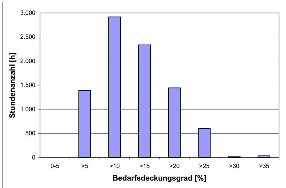
Abbildung 44: Häufigkeitsverteilung des aktuellen Bedarfsdeckungsgrades aus Wasserkraft bezogen auf den stündlichen Strombedarf (2005) in der Region Bruck an der Mur / Kapfenberg
