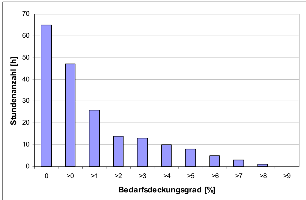
Abbildung 46: Repräsentative Häufigkeitsverteilung des Bedarfsdeckungsgrades der Solarstromerzeugung auf Stundenbasis in der Region Bruck an der Mur / Kapfenberg
