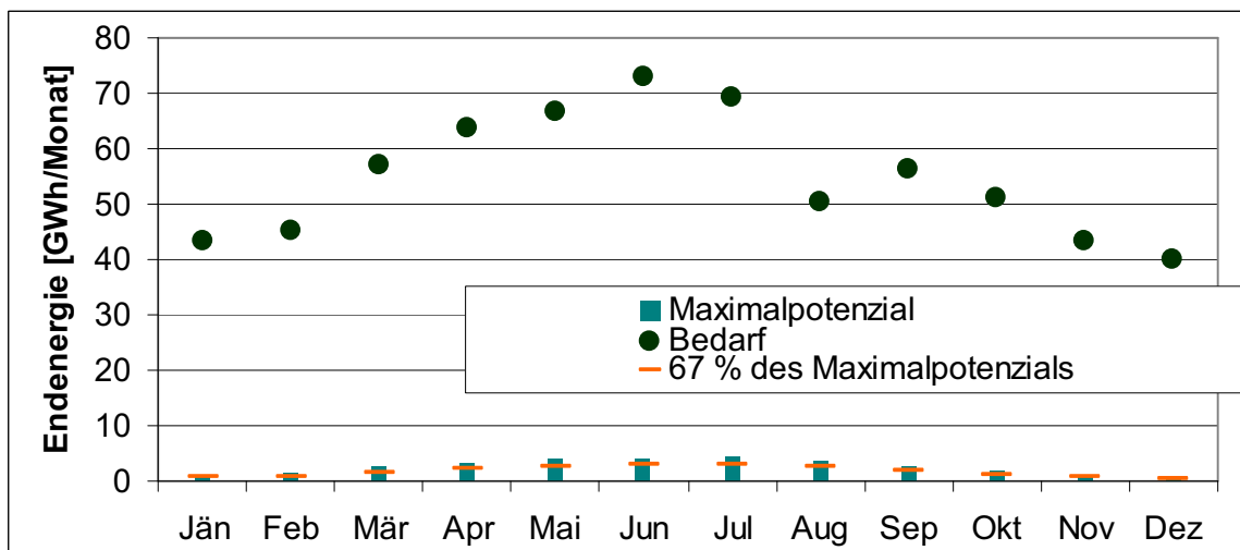
Abbildung 74: Monatlicher Strombedarf bei Tageslicht und monatliche Bereitstellung an Solarstrom mit einem photovoltaischen Deckungsgrad von 100 % sowie 67 % unter Berücksichtigung der thermischen Abfallverwertung und Umgebungswärme in der Niedertemperaturwärmebereitstellung in der Industrieregion Bruck an der Mur / Kapfenberg
