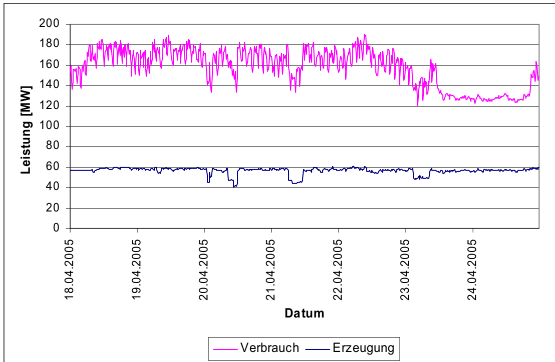
Abbildung 51: Leistungswerte der Stromerzeugung und des –verbrauches in der 3. Aprilwoche 2005 (Montag bis Sonntag) in der Modellregion (auf Basis von Viertelstundenwerten) [Beteiligte Firmen]
