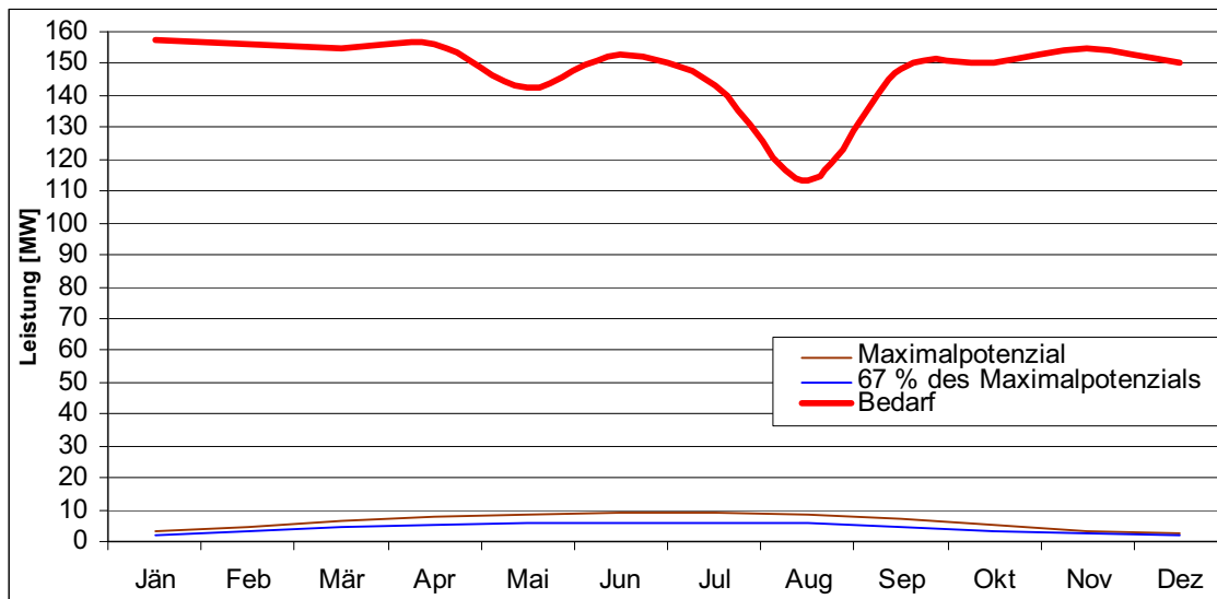
Abbildung 75: Mittlerer Leistungsbedarf an Strom und mittlere Leistungsbereitstellung an Solarstrom bei Tageslicht mit einem photovoltaischen Deckungsgrad von 100 % sowie 67 % im Jahresverlauf unter Berücksichtigung der thermischen Abfallverwertung und Umgebungswärme in der Niedertemperaturwärmebereitstellung in der Industrieregion Bruck an der Mur / Kapfenberg [Beteiligte Firmen], [Statistik Austria]; [E-Control 2]
