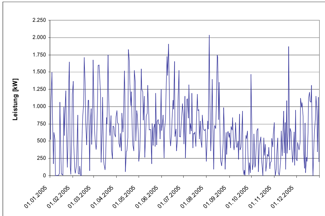
Abbildung 26: Synthetischer Jahrgang der Leistung einer möglichen Windenergieanlage (Enercon; 2MW) am Standort Mittagkogel auf Basis von Messungen in den Jahren 2000 und 2001 (Tagesmittelwerte)
