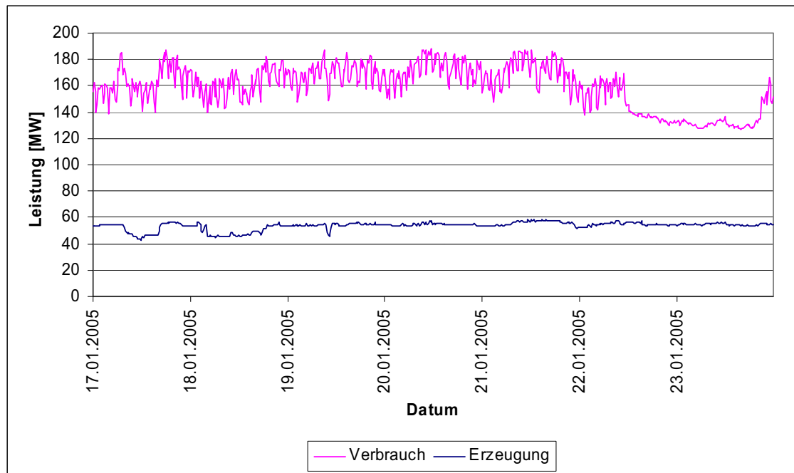
Abbildung 9: Leistungswerte der Stromerzeugung und des Stromverbrauches in der 3. Jännerwoche 2005 (Montag bis Sonntag) in der Modellregion (auf Basis von Viertelstundenwerten) [Beteiligte Firmen]
