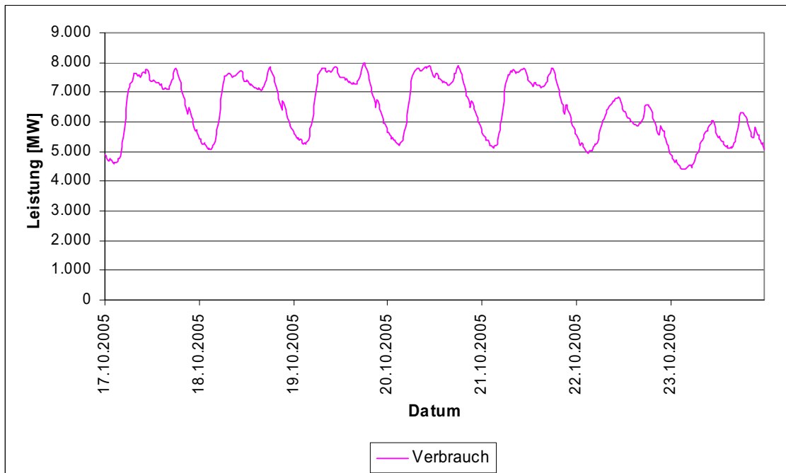
Abbildung 58: Leistungswerte des Stromverbrauches in der 3. Oktoberwoche 2005 (Montag bis Sonntag) in Österreich (auf Basis von Viertelstundenwerten) [E-Control 1, 2007]
