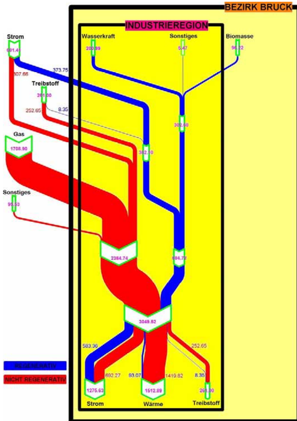
Abbildung 42: Ist-Situation der Energieflüsse in der Region auf Basis Endenergie
