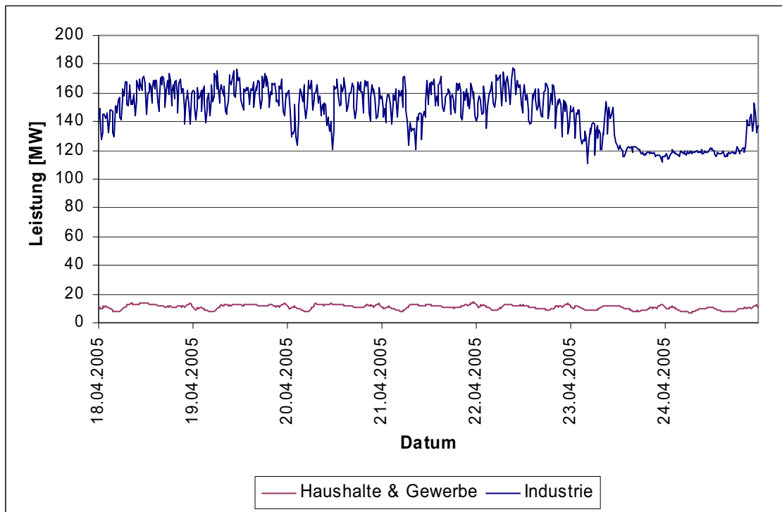
Abbildung 50: Leistungswerte des Stromverbrauches der 3. Aprilwoche 2005 (Montag bis Sonntag) nach Sektoren in der Modellregion (auf Basis von Viertelstundenwerten) [Beteiligte Firmen]
