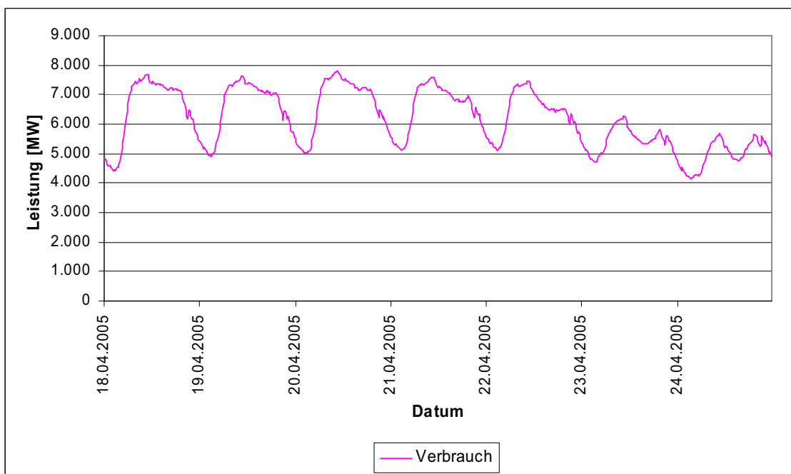
Abbildung 52: Leistungswerte des Stromverbrauches in der 3. Aprilwoche 2005 (Montag bis Sonntag) in Österreich (auf Basis von Viertelstundenwerten) [E-Control 1, 2007]
