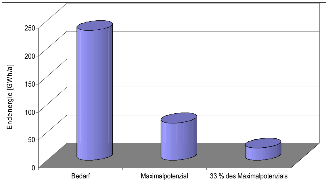
Abbildung 70: Jährlicher Wärmeverbrauch der Haushalte und jährliche Solarwärmeerzeugung mit einem solarthermischen Deckungsgrad von 100 % sowie 33 % in der Industrieregion Bruck an der Mur / Kapfenberg
