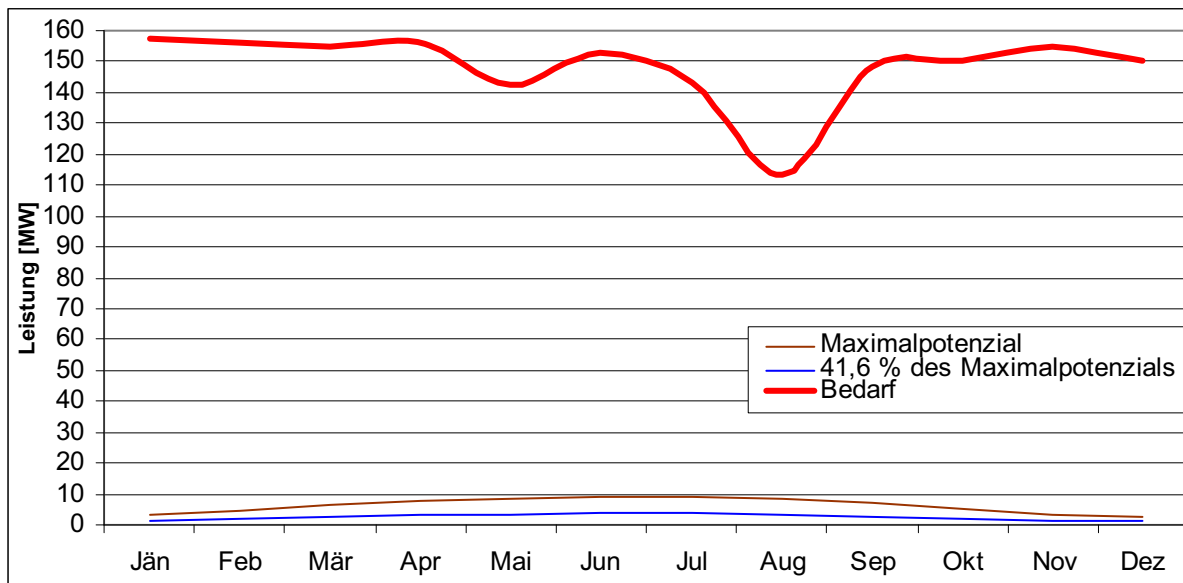
Abbildung 39: Mittlerer Leistungsbedarf an Strom und mittlere Leistungsbereitstellung an Solarstrom bei Tageslicht mit einem photovoltaischen Deckungsgrad von 100 % sowie 41,6 % im Jahresverlauf in der Industrieregion Bruck an der Mur / Kapfenberg [Beteiligte Firmen], [Statistik Austria]; [E-Control 2]
