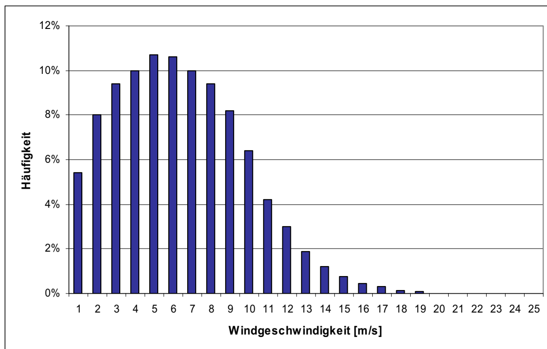
Abbildung 25: Verteilung der Windgeschwindigkeiten am Standort Mittagkogel auf Basis von Halbstundenwerten
