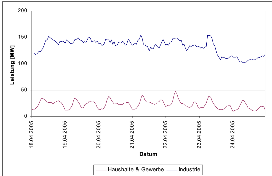
Abbildung 59: Leistung des Erdgasverbrauches der 3. Aprilwoche 2005 (Montag bis Sonntag) nach Sektoren in der Industrieregion Bruck an der Mur / Kapfenberg (auf Basis von Stundenwerten) [Beteiligte Firmen]
