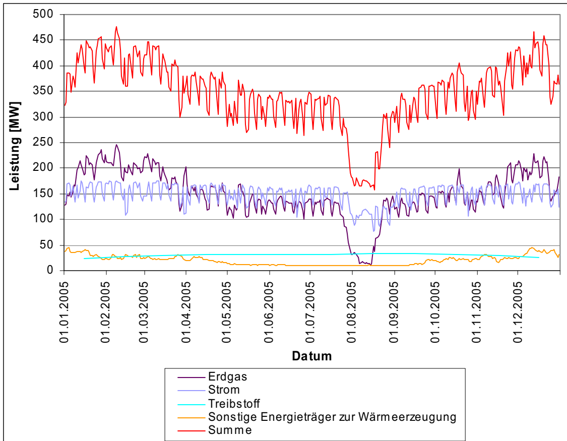
Abbildung 20: Mittlere Tagesleistung des Verbrauches an betrachteten Endenergieträgern im Jahresverlauf in der Modellregion [Beteiligte Firmen]
