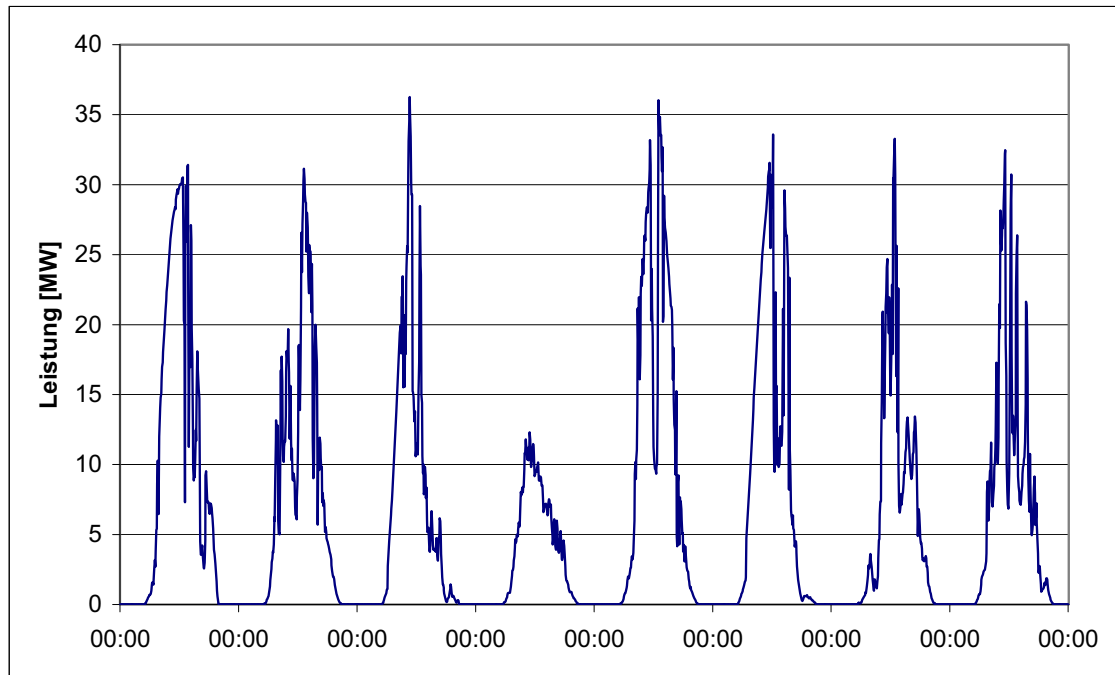
Abbildung 35: Repräsentativer potenzieller Leistungsverlauf an Solarthermie in der Industrieregion Bruck an der Mur / Kapfenberg
