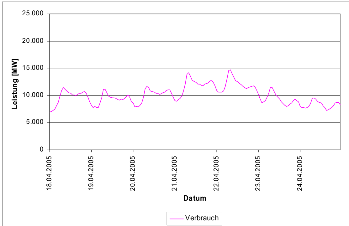
Abbildung 60: Leistung des Erdgasverbrauches der 3. Aprilwoche 2005 (Montag bis Sonntag) in Österreich (auf Basis von Stundenwerten) [E-Control 2, 2007]
