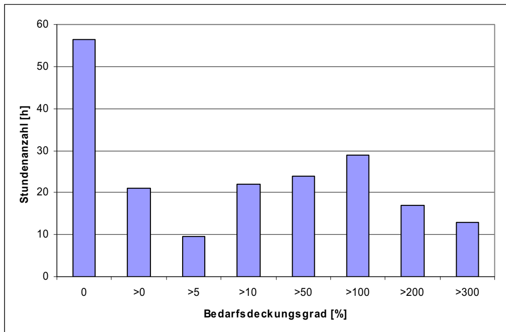
Abbildung 47: Repräsentative Häufigkeitsverteilung des Bedarfsdeckungsgrades der Solarwärmeerzeugung auf Stundenbasis in der Region Bruck an der Mur / Kapfenberg
