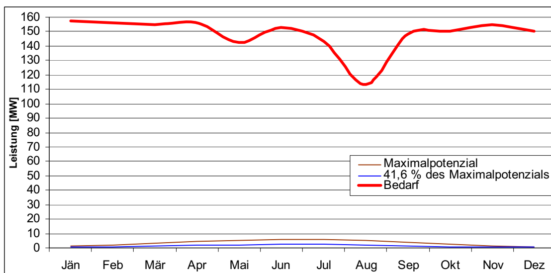
Abbildung 37: Mittlerer täglicher Leistungsbedarf an Strom und mittlere tägliche Leistungsbereitstellung an Solarstrom mit einem photovoltaischen Deckungsgrad von 100 % sowie 41,6 % im Jahresverlauf in der Industrieregion Bruck an der Mur / Kapfenberg [Beteiligte Firmen], [Statistik Austria 2, 2001], [Statistik Austria 3, 2001], [Statistik Austria 5, 2007]
