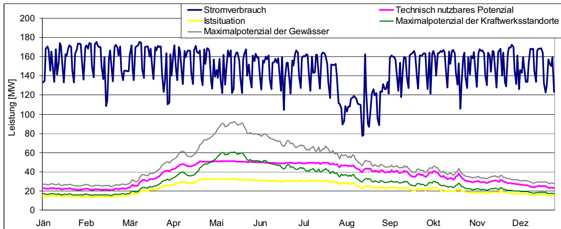
Abbildung 31: Gesamtstromverbrauch des Jahres 2005 der Region Bruck an der Mur / Kapfenberg sowie aktuelle Leistung der Wasserkraftwerke bzw. bei unterschiedlichen Szenarien [Tagesmittelwerte]
