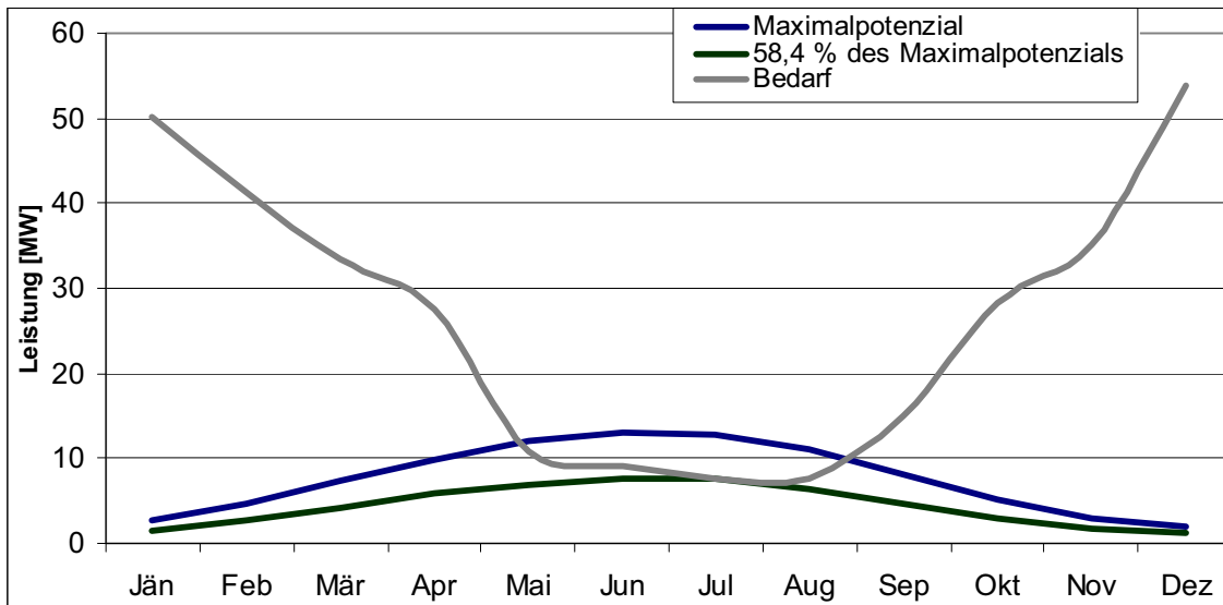
Abbildung 34: Mittlerer täglicher Leistungsbedarf an Wärme der Haushalte und mittlere tägliche Leistungsbereitstellung an Solarwärme mit einem solarthermischen Deckungsgrad von 100 % sowie 58,4 % im Jahresverlauf in der Industrieregion Bruck an der Mur / Kapfenberg [Beteiligte Firmen], [Statistik Austria 2, 2001], [Statistik Austria 3, 2001], [Statistik Austria 5, 2007]
