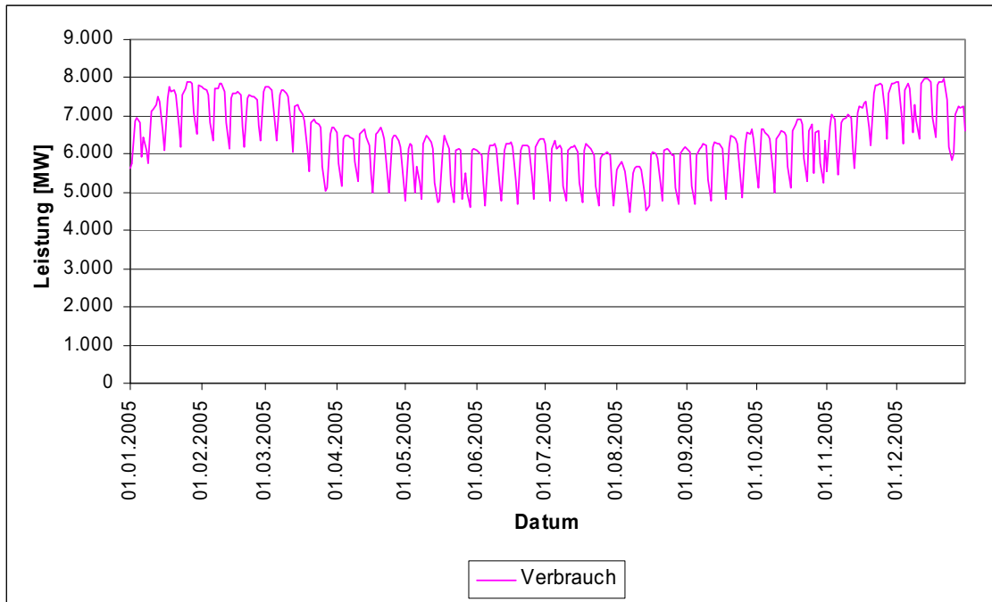
Abbildung 5: Mittlere Tagesleistung des Stromverbrauches im Jahresverlauf in Österreich 2005 (ohne Verbrauch für Pumpspeicherung) [E-Control 1, 2007]
