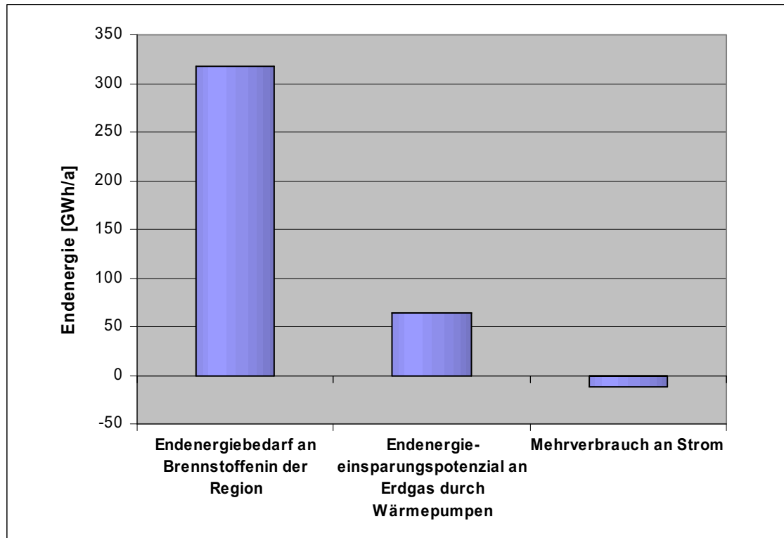
Abbildung 41: Endenergiebedarf an Brennstoffen, Endenergieeinsparungspotenzial und Mehrverbrauch an Strom durch Wärmepumpenanwendungen in der Industrieregion Bruck an der Mur / Kapfenberg
