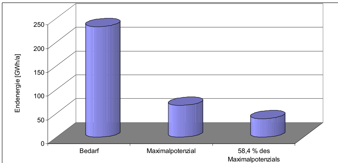
Abbildung 33: Jährlicher Wärmeverbrauch der Haushalte und jährliche Solarwärmeerzeugung mit einem solarthermischen Deckungsgrad von 100 % sowie 58,4 % in der Industrieregion Bruck an der Mur / Kapfenberg
