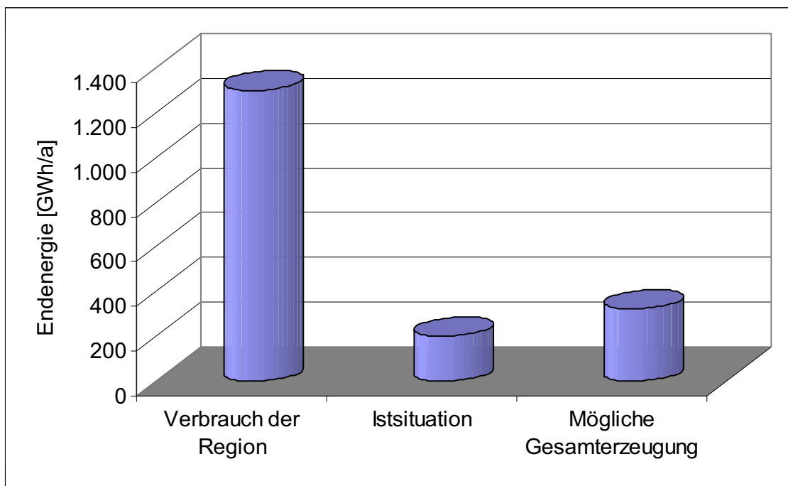
Abbildung 30: Gesamtstromverbrauch des Jahres 2005, Ist-Situation sowie mögliche Gesamterzeugung der Wasserkraft in der Region Bruck an der Mur / Kapfenberg [Beteiligte Firmen], [BMLFUW, 2007], [BH Bruck a. d. Mur, 2007], [Giesecke, 2005], [König, 2005]
