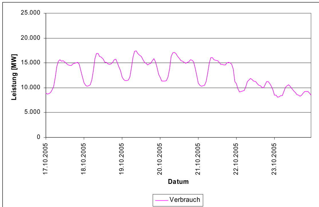
Abbildung 64: Leistung des Erdgasverbrauches der 3. Oktoberwoche 2005 (Montag bis Sonntag) in Österreich (auf Basis von Stundenwerten) [E-Control 2, 2007]
