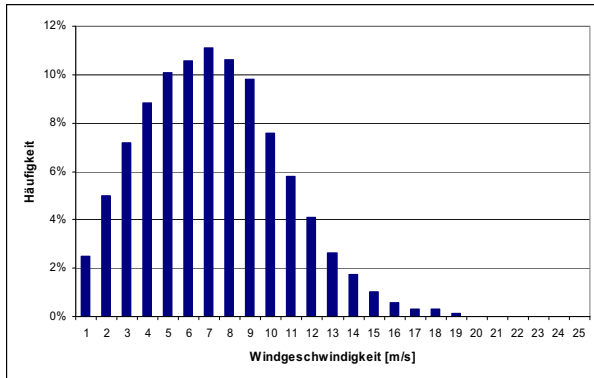
Abbildung 65: Verteilung der Windgeschwindigkeiten am Standort Dornerkogel auf Basis von Halbstundenwerten
