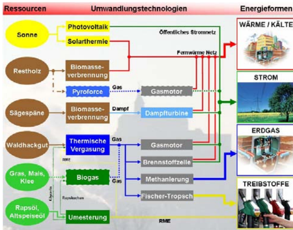
Abbildung 23: Energiesystem in der Stadt Güssing [Koch, 2006]
