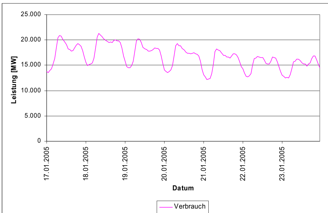
Abbildung 14: Mittlere Leistung des Gasverbrauches der 3. Jännerwoche 2005 (Montag bis Sonntag) in Österreich (auf Basis von Stundenwerten) [E-Control 2, 2007]
