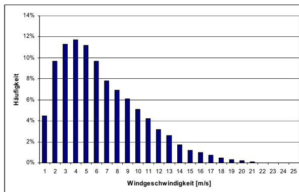
Abbildung 69: Verteilung der Windgeschwindigkeiten am Standort Predigtstuhl auf Basis von Halbstundenwerten
