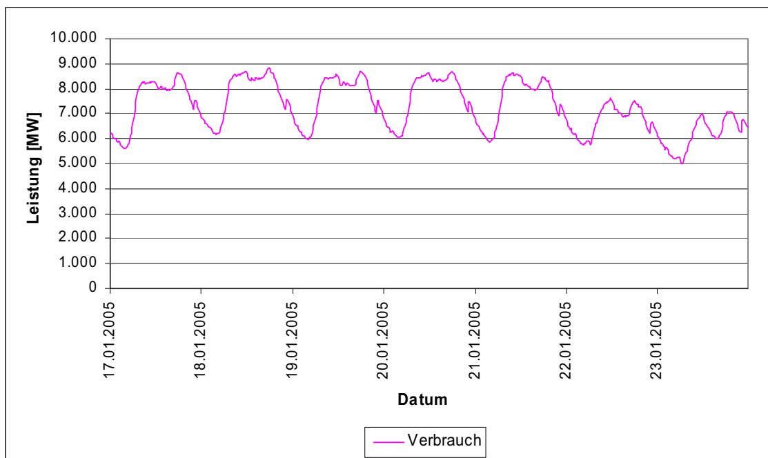
Abbildung 8: Leistungswerte des Stromverbrauches in der 3. Jännerwoche 2005 (Montag bis Sonntag) in Österreich (auf Basis von Viertelstundenwerten) [E-Control 1, 2007]
