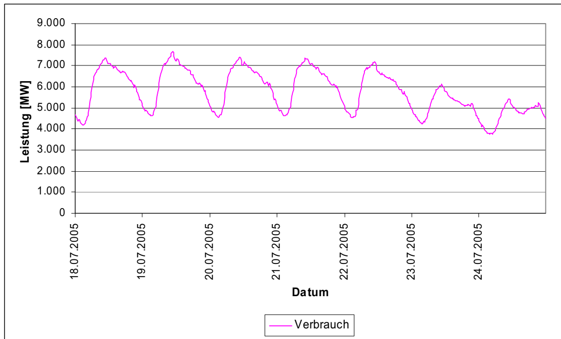
Abbildung 55: Leistungswerte des Stromverbrauches in der 3. Juliwoche 2005 (Montag bis Sonntag) in Österreich (auf Basis von Viertelstundenwerten) [E-Control 1, 2007]
