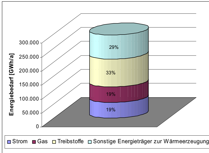
Abbildung 19: Anteil der betrachteten Energieträger am energetischen Endverbrauch in Österreich im Jahr 2005 [Statistik Austria 1, 2005]
