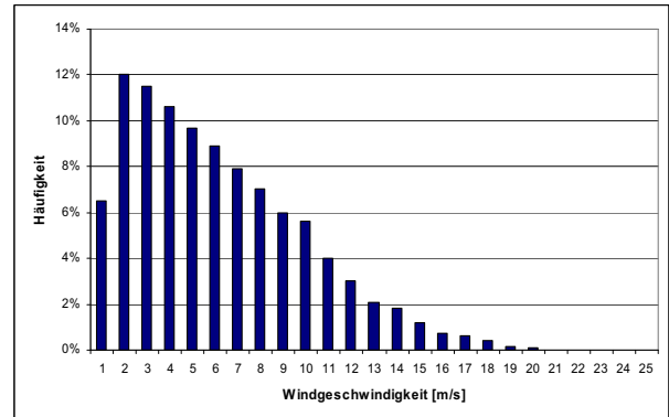
Abbildung 67: Verteilung der Windgeschwindigkeiten am Standort Zöberer Höhe auf Basis von Halbstundenwerten
