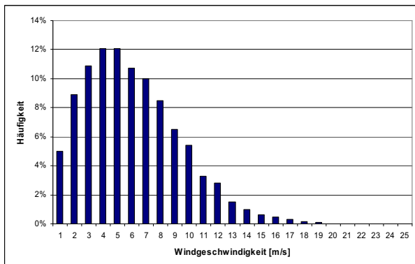
Abbildung 66: Verteilung der Windgeschwindigkeiten am Standort Schwarzkogel auf Basis von Halbstundenwerten
