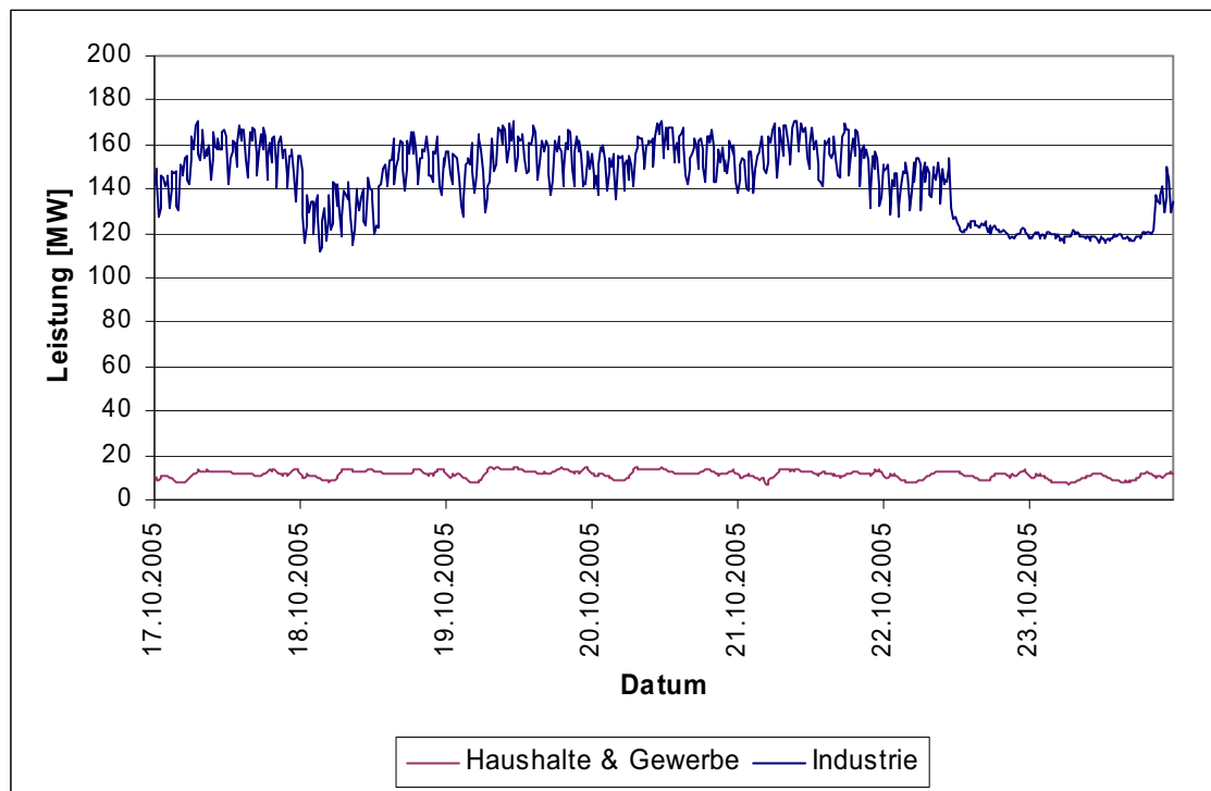
Abbildung 56: Leistungswerte des Stromverbrauches der 3. Oktoberwoche 2005 (Montag bis Sonntag) nach Sektoren in der Modellregion (auf Basis von Viertelstundenwerten) [Beteiligte Firmen]
