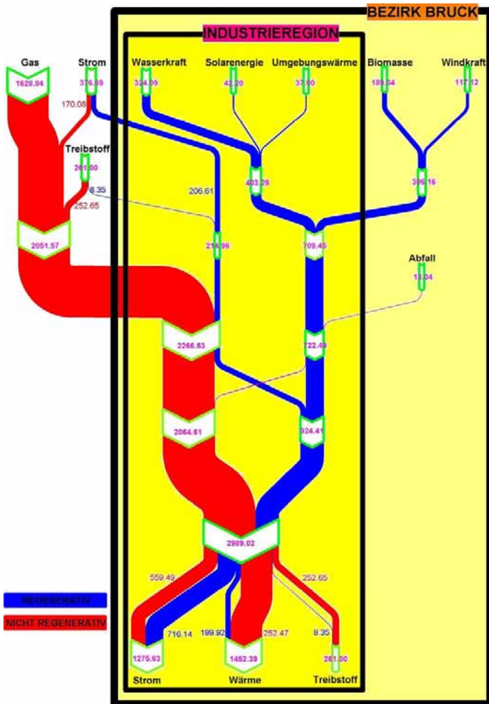
Abbildung 49: Szenario der Energieflüsse in der Region auf Basis von Endenergie
