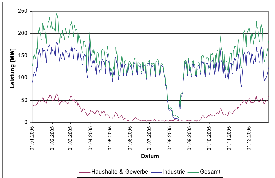
Abbildung 11: Mittlere Tagesleistung des Erdgasverbrauches im Jahresverlauf (2005) nach Sektoren in der Industrieregion Bruck an der Mur / Kapfenberg [Beteiligte Firmen]
