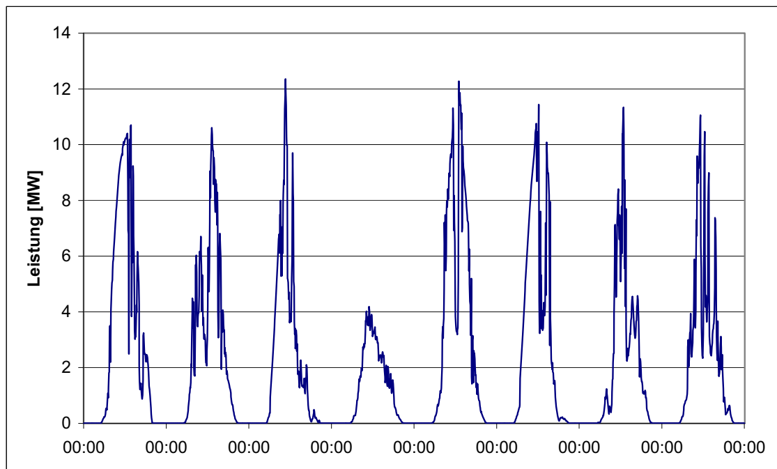
Abbildung 40: Repräsentativer potenzieller Leistungsverlauf an Solarstrombereitstellung in der Industrieregion Bruck an der Mur / Kapfenberg
