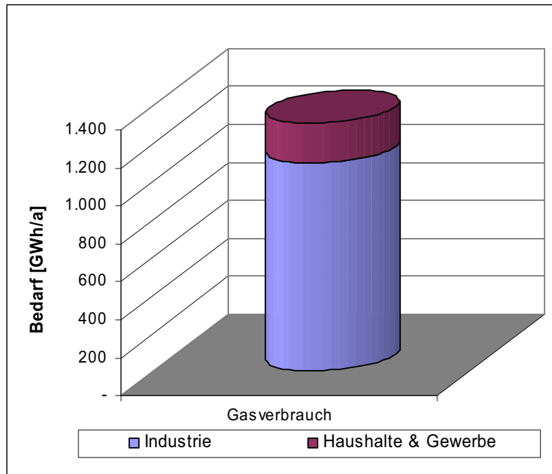
Abbildung 10: Bedarf an Erdgas als Endenergieträger in der Industrieregion (Bedarf an Erdgas als Sekundärenergieträger nicht berücksichtigt) [Beteiligte Firmen]
