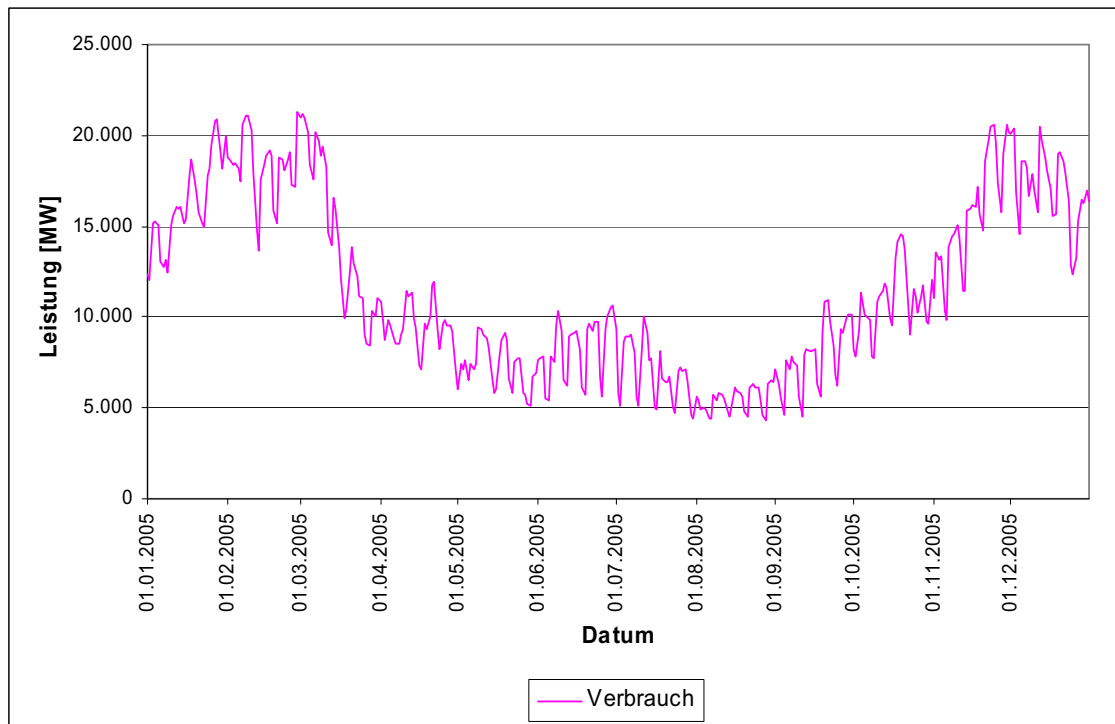
Abbildung 12: Mittlere Tagesleistung des Erdgasverbrauches im Jahresverlauf (2005) in Österreich [E-Control 2, 2007]
