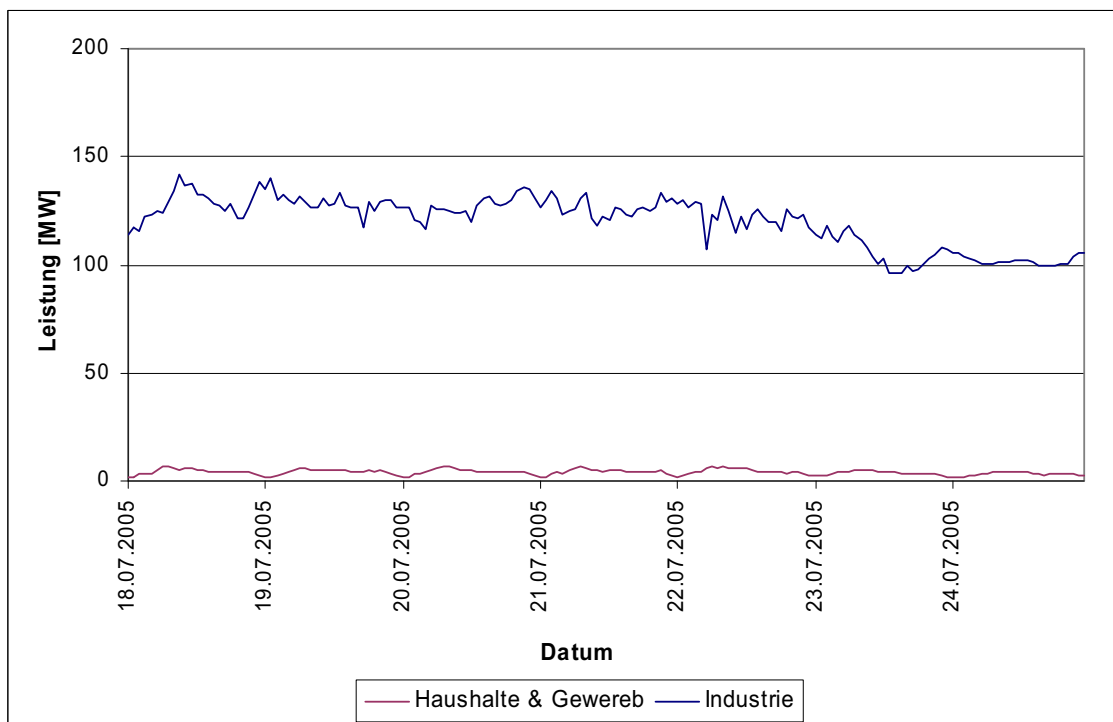
Abbildung 61: Leistung des Erdgasverbrauches der 3. Juliwoche 2005 (Montag bis Sonntag) nach Sektoren in der Industrieregion Bruck an der Mur / Kapfenberg (auf Basis von Stundenwerten) [Beteiligte Firmen]
