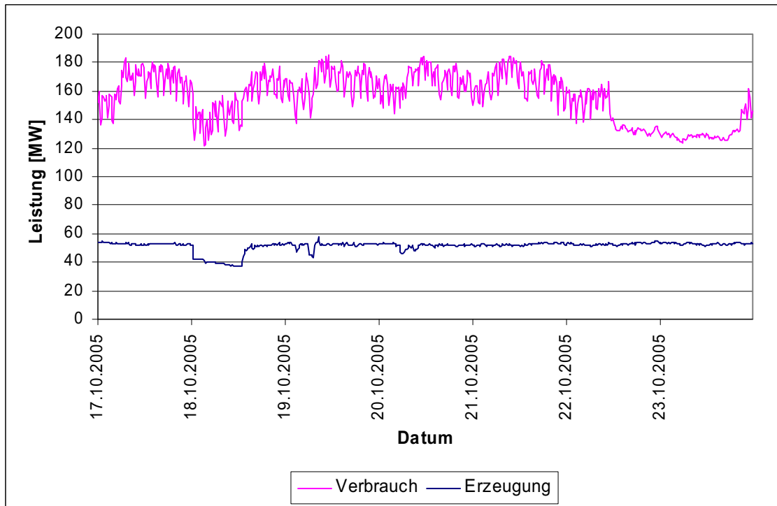
Abbildung 57: Leistungswerte der Stromerzeugung und des –verbrauches in der 3. Oktoberwoche 2005 (Montag bis Sonntag) in der Modellregion (auf Basis von Viertelstundenwerten) [Beteiligte Firmen]
