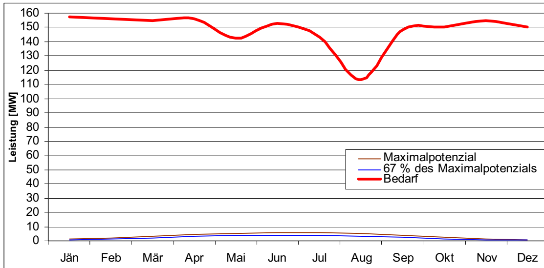
Abbildung 73: Mittlerer täglicher Leistungsbedarf an Strom und mittlere tägliche Leistungsbereitstellung an Solarstrom mit einem photovoltaischen Deckungsgrad von 100 % sowie 67 % im Jahresverlauf unter Berücksichtigung der thermischen Abfallverwertung und Umgebungswärme in der Niedertemperaturwärmebereitstellung in der Industrieregion Bruck an der Mur / Kapfenberg
