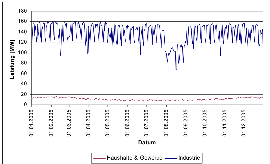
Abbildung 4: Mittlere Tagesleistung des Stromverbrauches im Jahresverlauf (2005) nach Sektoren in der Modellregion [Beteiligte Firmen]
