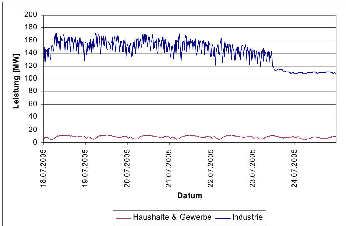
Abbildung 53: Leistungswerte des Stromverbrauches der 3. Juliwoche 2005 (Montag bis Sonntag) nach Sektoren in der Modellregion (auf Basis von Viertelstundenwerten) [Beteiligte Firmen]
