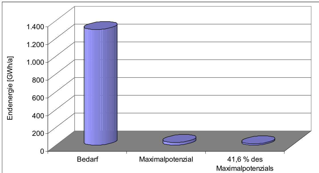
Abbildung 36: Jährlicher Gesamtstromverbrauch und jährliche Solarstromerzeugung mit einem photovoltaischen Deckungsgrad von 100 % sowie 41,6 % in der Industrieregion Bruck an der Mur / Kapfenberg [Beteiligte Firmen], [Statistik Austria 2, 2001], [Statistik Austria 3, 2001], [Statistik Austria 5, 2007]
