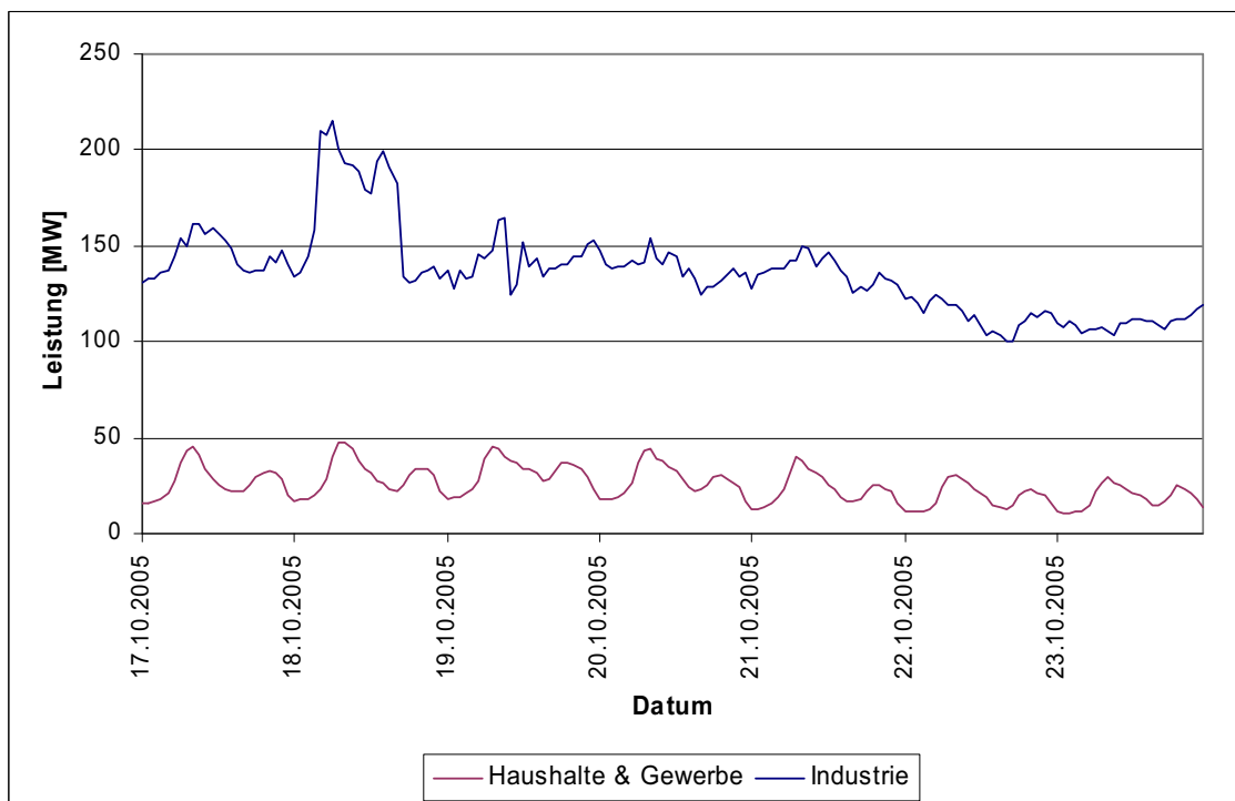
Abbildung 63: Leistung des Erdgasverbrauches der 3. Oktoberwoche 2005 (Montag bis Sonntag) nach Sektoren in der Industrieregion Bruck an der Mur / Kapfenberg (auf Basis von Stundenwerten) [Beteiligte Firmen]
