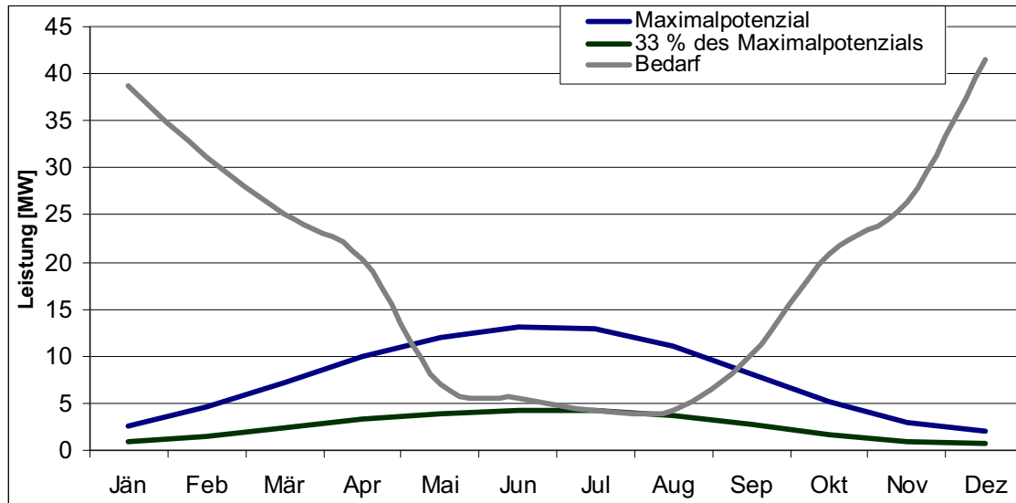
Abbildung 71: Mittlerer täglicher Leistungsbedarf an Wärme der Haushalte und mittlere tägliche Leistungsbereitstellung an Solarwärme mit einem solarthermischen Deckungsgrad von 100 % sowie 33 % im Jahresverlauf in der Industrieregion Bruck an der Mur / Kapfenberg [Beteiligte Firmen], [Statistik Austria 2, 2001], [Statistik Austria 3, 2001], [Statistik Austria 5, 2007]
