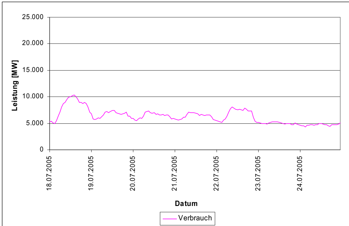
Abbildung 62: Leistung des Erdgasverbrauches der 3. Juliwoche 2005 (Montag bis Sonntag) in Österreich (auf Basis von Stundenwerten) [E-Control 2, 2007]
