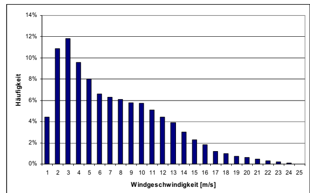
Abbildung 68: Verteilung der Windgeschwindigkeiten am Standort Wohntalhocheck auf Basis von Halbstundenwerten
