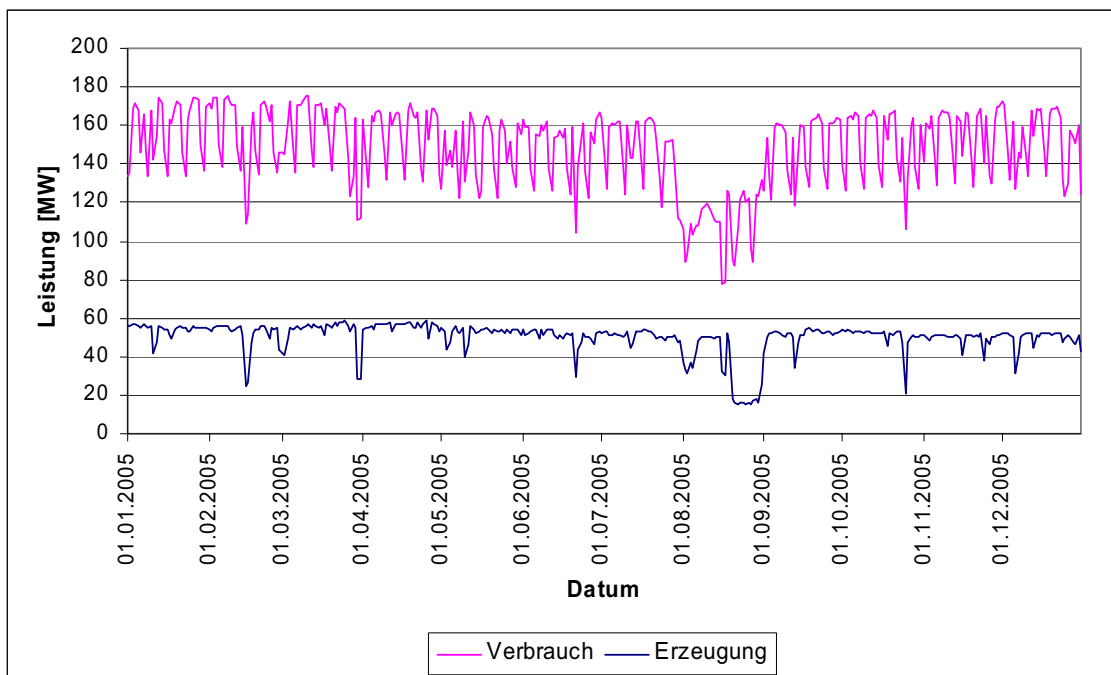
Abbildung 6: Mittlere Tagesleistung der Stromerzeugung und des Stromverbrauches im Jahresverlauf (2005) in der Modellregion [Beteiligte Firmen]
