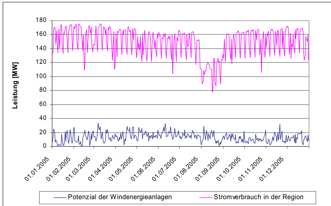
Abbildung 29: Gegenüberstellung der Stromerzeugung aus Windkraft und Gesamtstromverbrauch der Region Bruck an der Mur / Kapfenberg im Jahresverlauf 2005 (Tagesmittelwerte) [Beteiligte Firmen]
