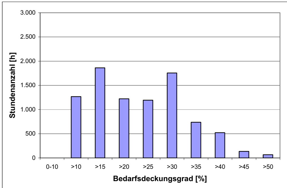
Abbildung 45: Häufigkeitsverteilung des potenziellen Bedarfsdeckungsgrades aus Wasserkraft bezogen auf den stündlichen Strombedarf (2005) in der Region Bruck an der Mur / Kapfenberg
