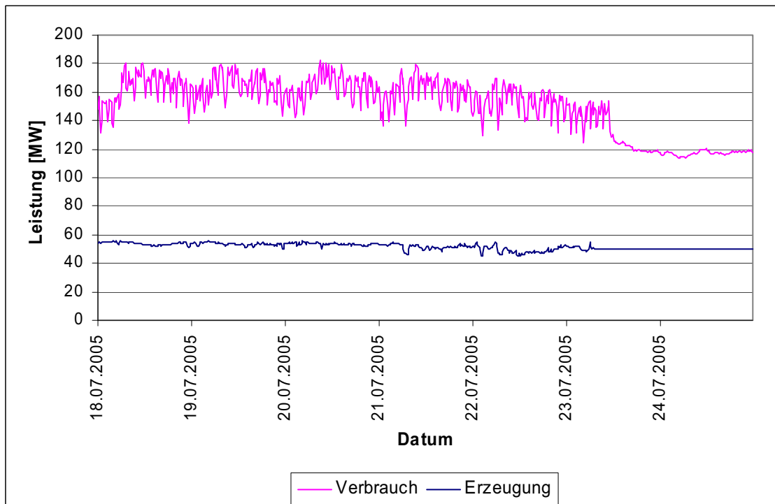
Abbildung 54: Leistungswerte der Stromerzeugung und des -verbrauches in der 3. Juliwoche 2005 (Montag bis Sonntag) in der Modellregion (auf Basis von Viertelstundenwerten) [Beteiligte Firmen]
