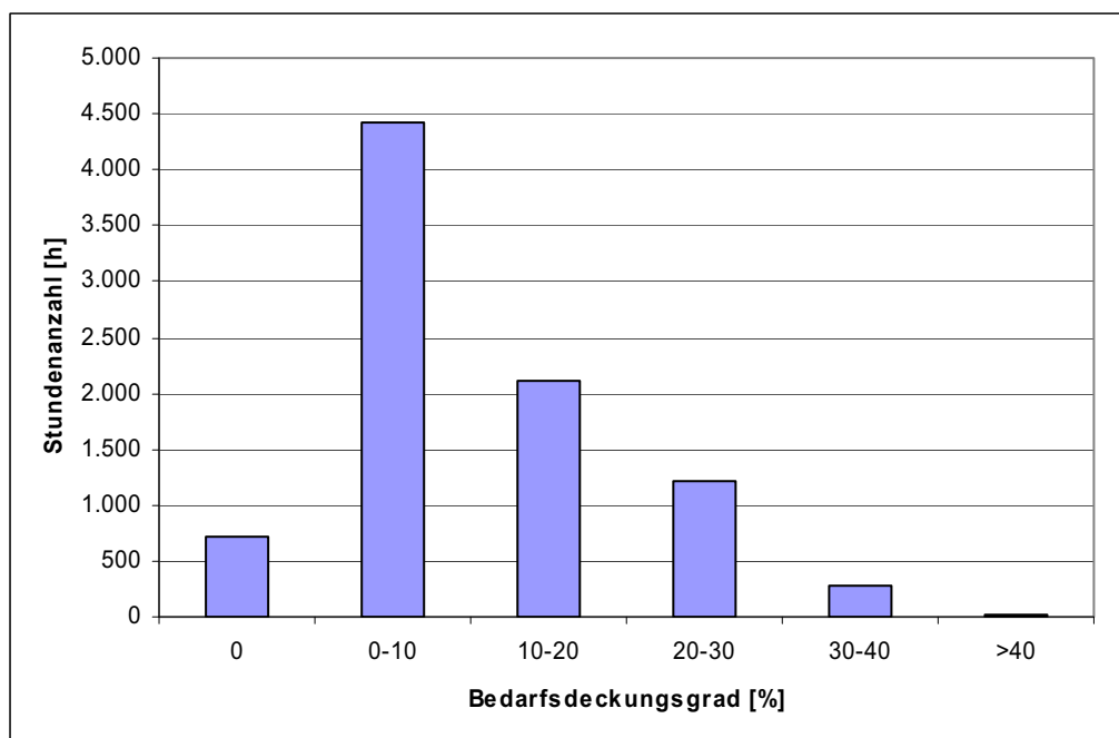
Abbildung 43: Häufigkeitsverteilung des Bedarfsdeckungsgrades der Windenergieerzeugung auf Stundenbasis in der Region Bruck an der Mur / Kapfenberg (2005)
