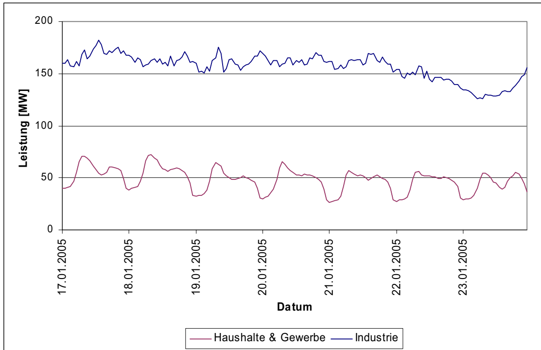
Abbildung 13: Mittlere Leistung des Gasverbrauches der 3. Jännerwoche 2005 (Montag bis Sonntag) nach Sektoren in der Industrieregion Bruck an der Mur / Kapfenberg (auf Basis von Stundenwerten) [Beteiligte Firmen]
