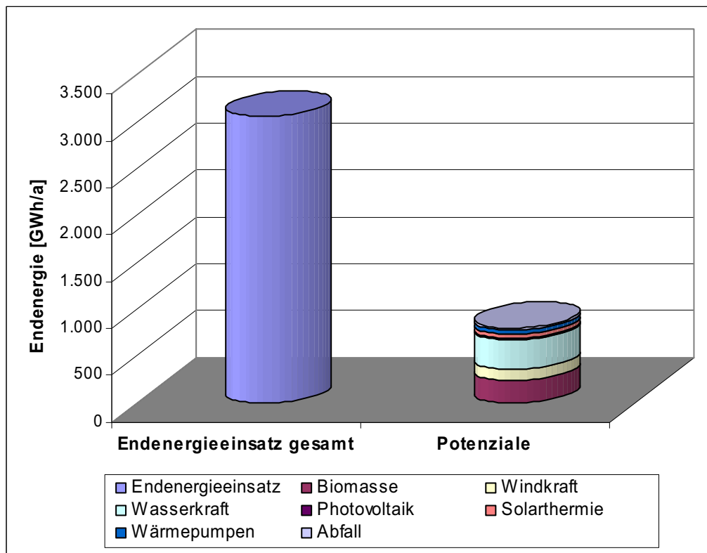
Abbildung 48: Potenzial erneuerbarer Energie inklusive Abfall im Vergleich mit dem Endenergieeinsatz in der Industrieregion Bruck an der Mur / Kapfenberg
