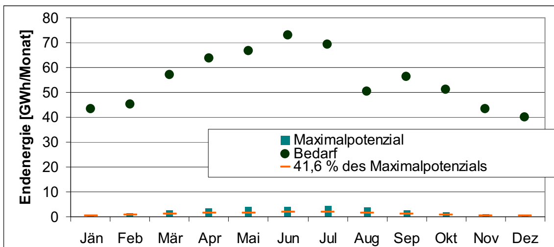
Abbildung 38: Monatlicher Strombedarf bei Tageslicht und monatliche Bereitstellung an Solarstrom mit einem photovoltaischen Deckungsgrad von 100 % sowie 41,6 % in der Industrieregion Bruck an der Mur / Kapfenberg
